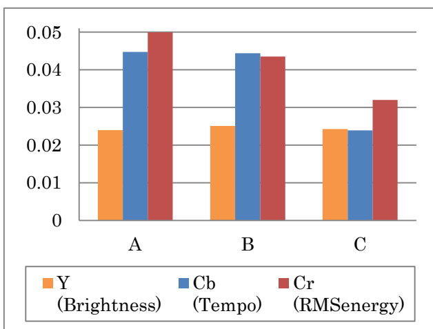
図 6. プレイリスト別の各特徴量の分散値
